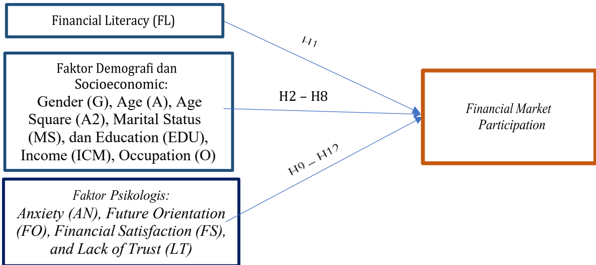
Gambar 1 Kerangka Penelitian
