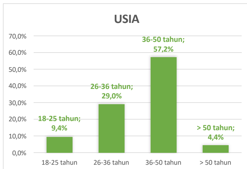
Gambar 2 Usia Responden
