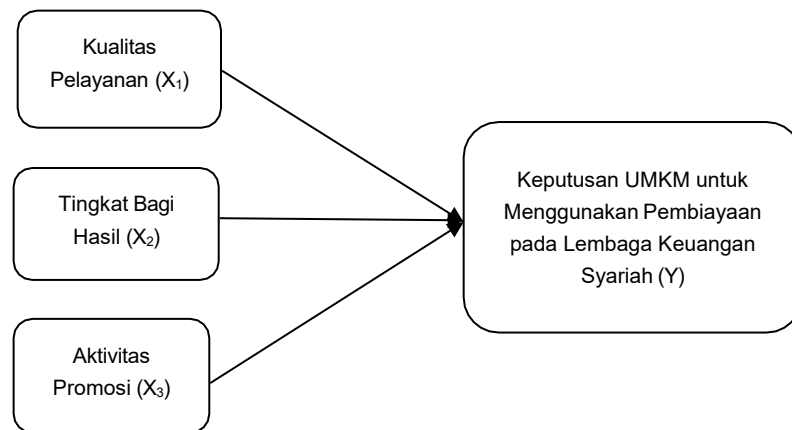
Gambar 1 Kerangka Pemikiran
