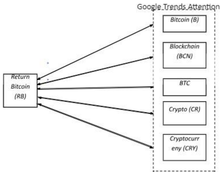
Gambar 2 Kerangka Pemikiran
