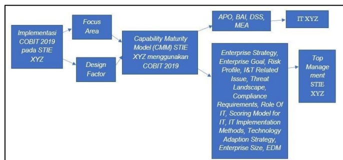
Gambar 5 Kerangka Pemikiran
